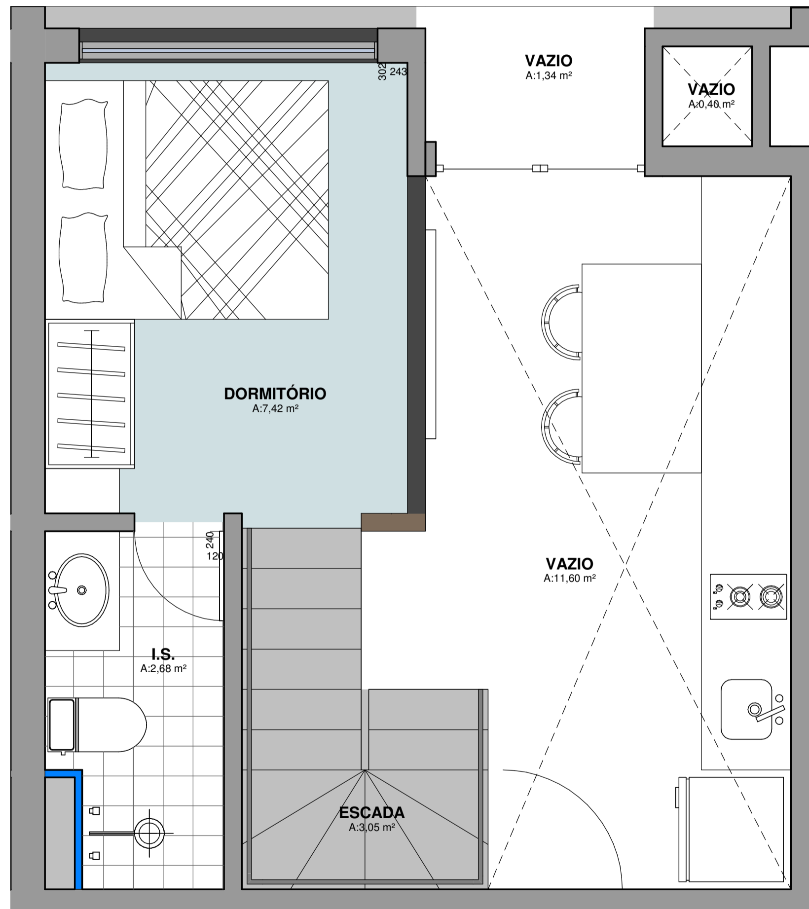
MEZANINO 107 ESCALA 1 : 25
