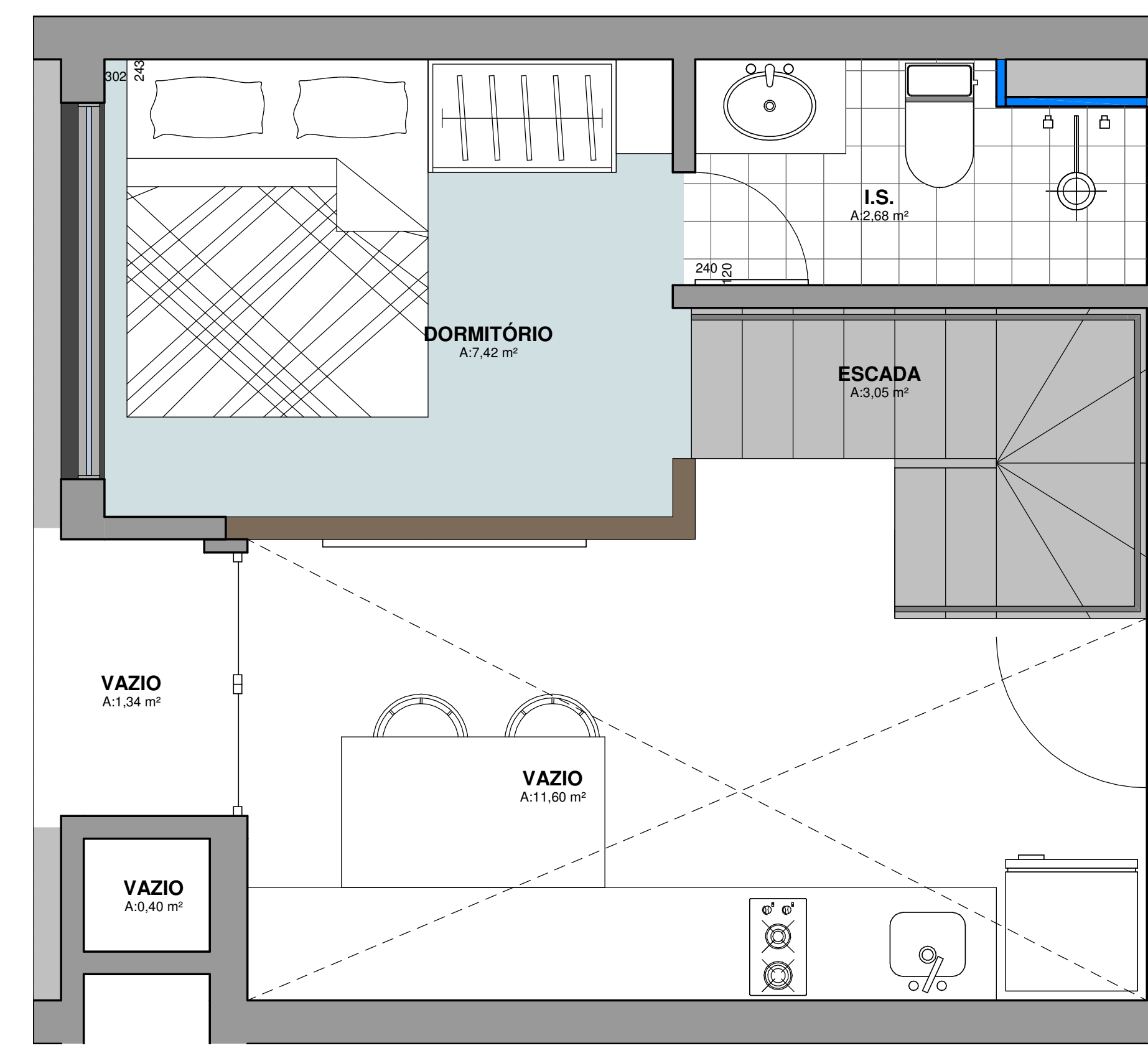
MEZANINO 110 ESCALA 1 : 25
