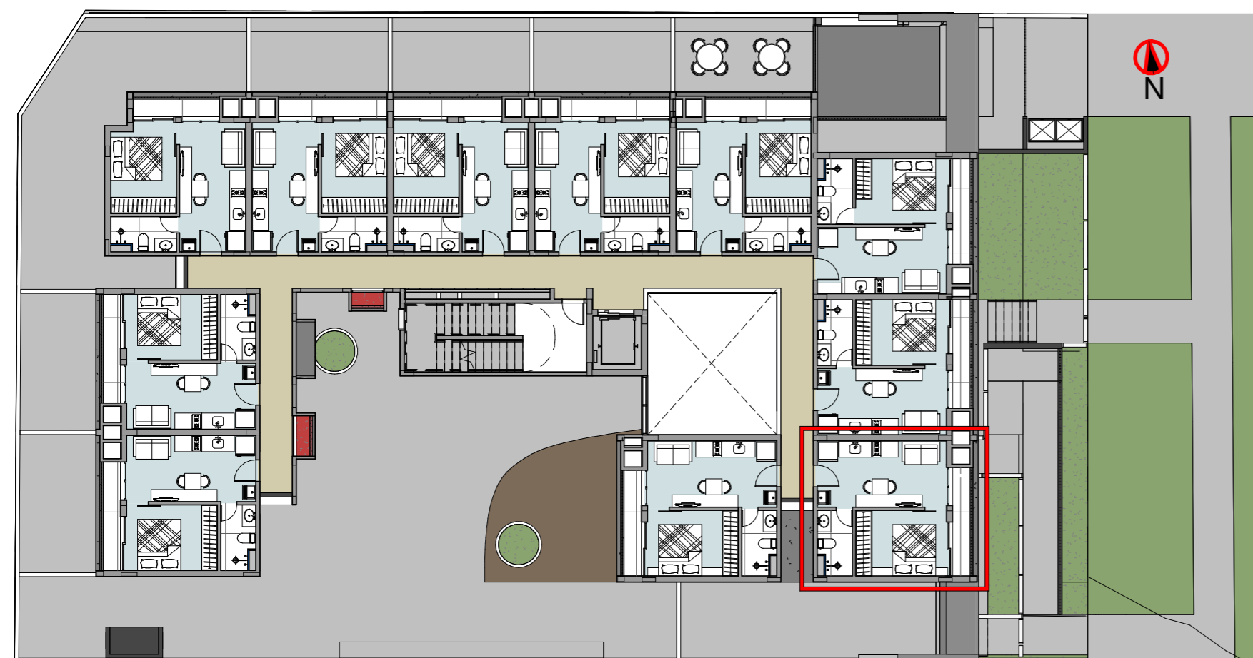
1 -PAVTO TIPO (2º,3º E 4º) ESCALA 1 : 200
