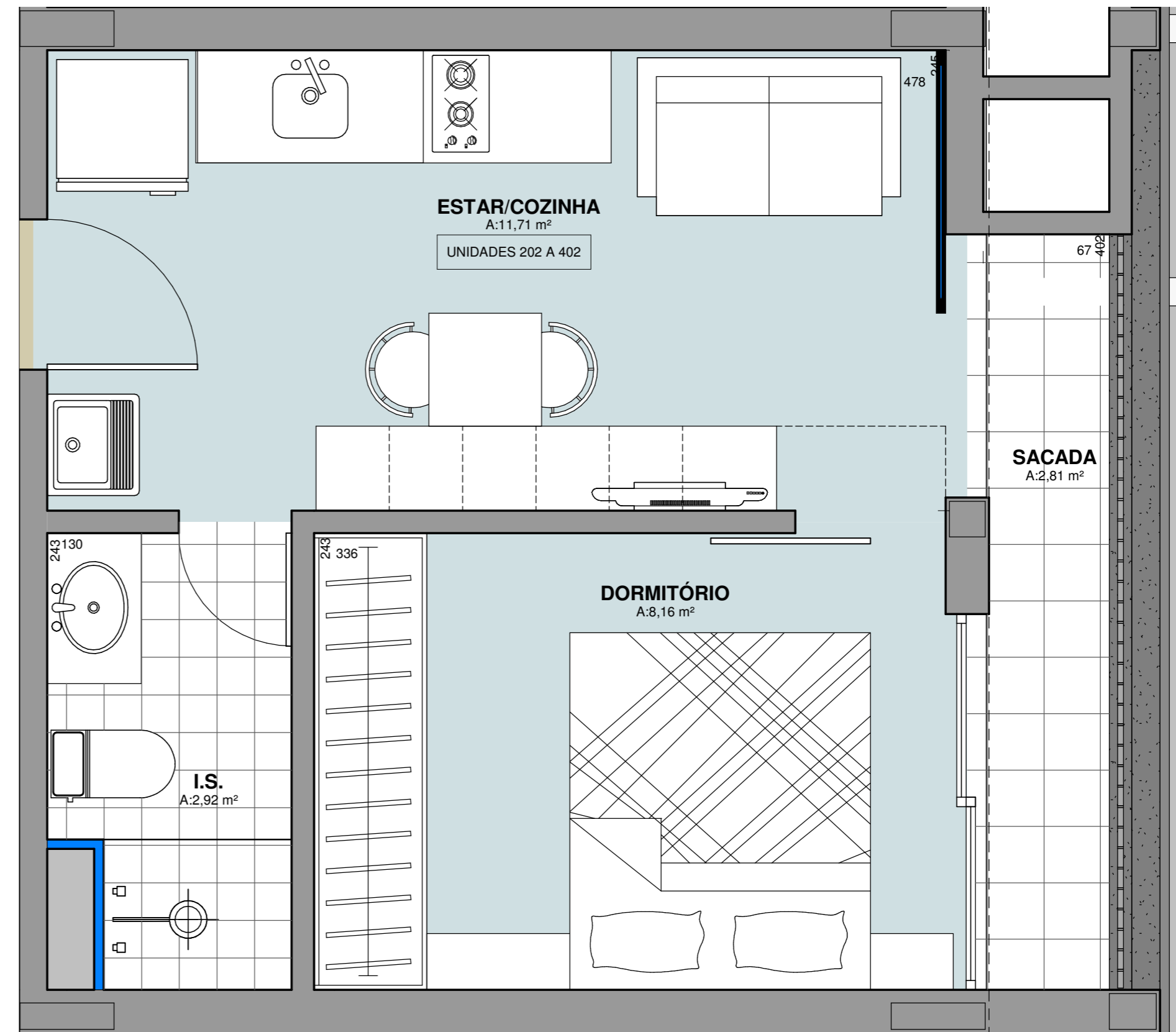
UNIDADE TIPO - 202 A 402 ESCALA 1 : 25
