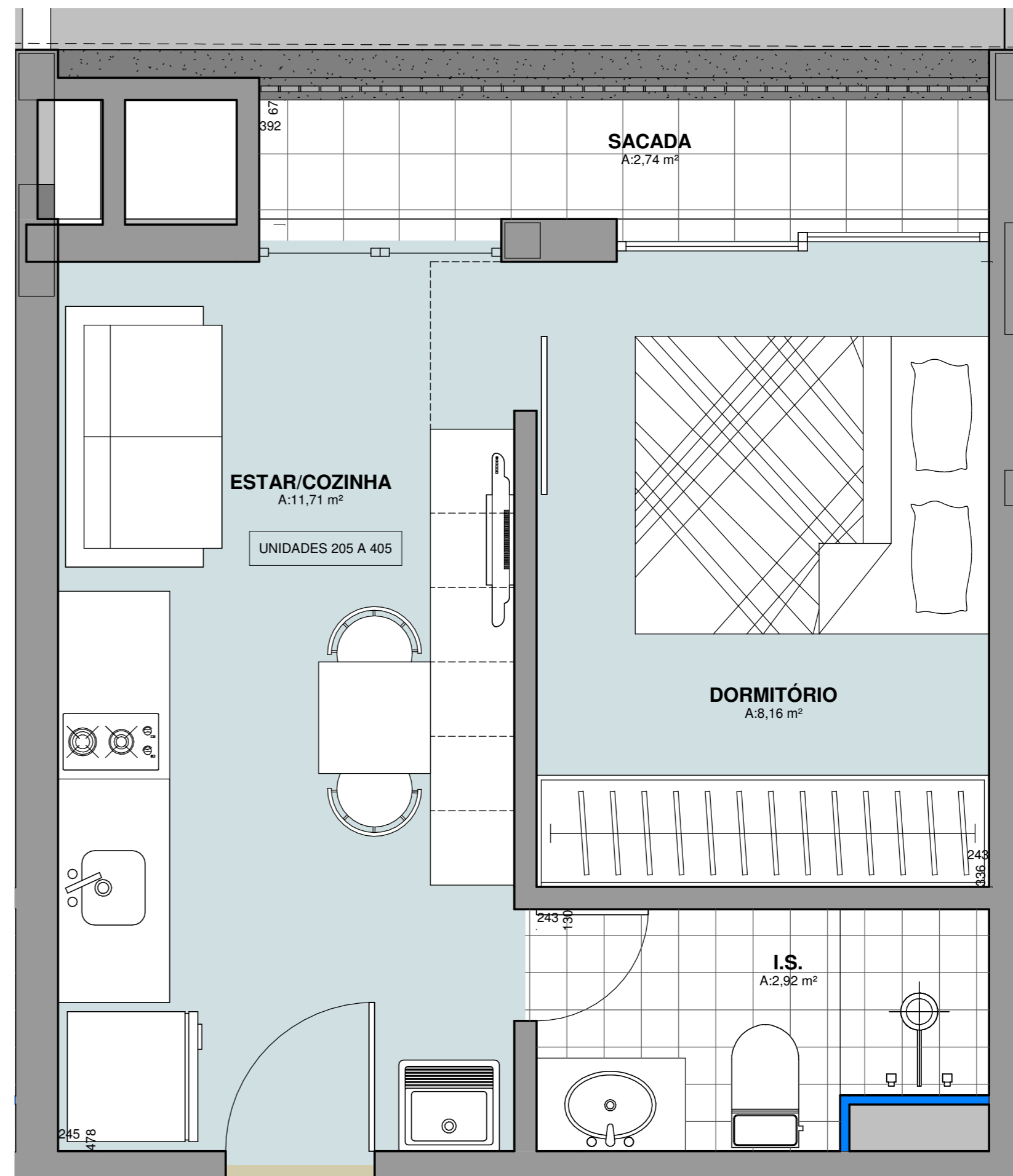
UNIDADE TIPO - 205 A 405
