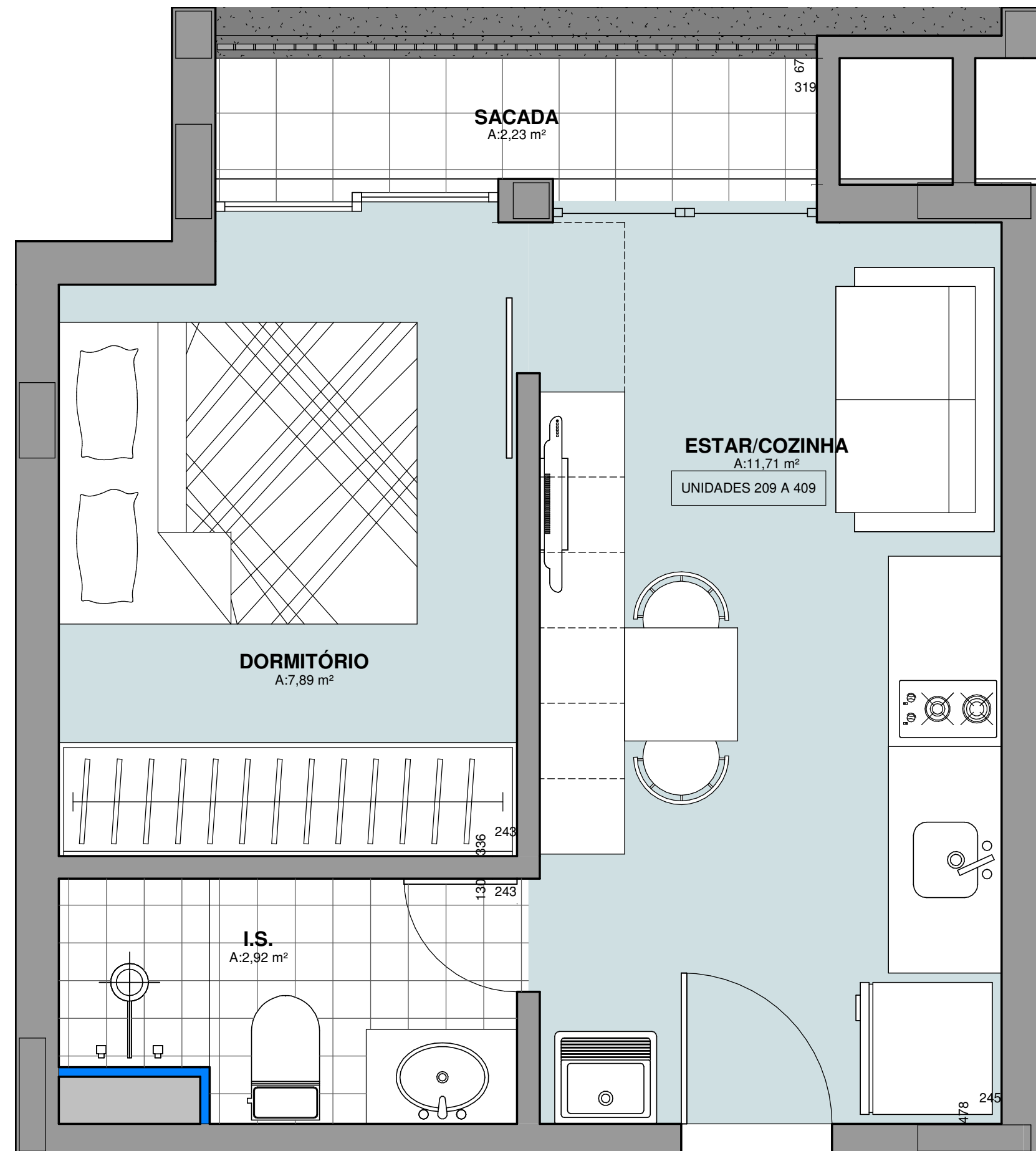
UNIDADE TIPO - 209 A 409 ESCALA 1 : 25
