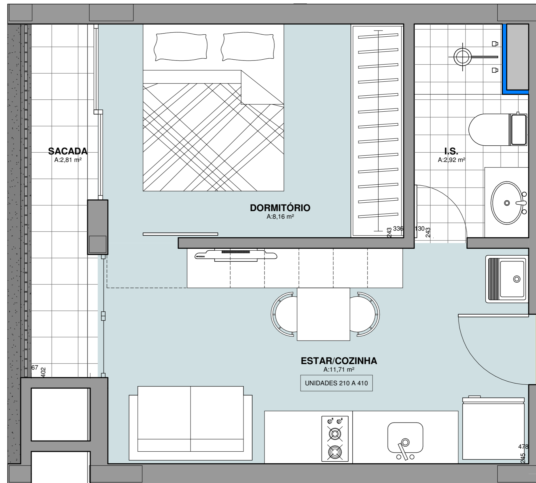
UNIDADE TIPO - 210 A 410
