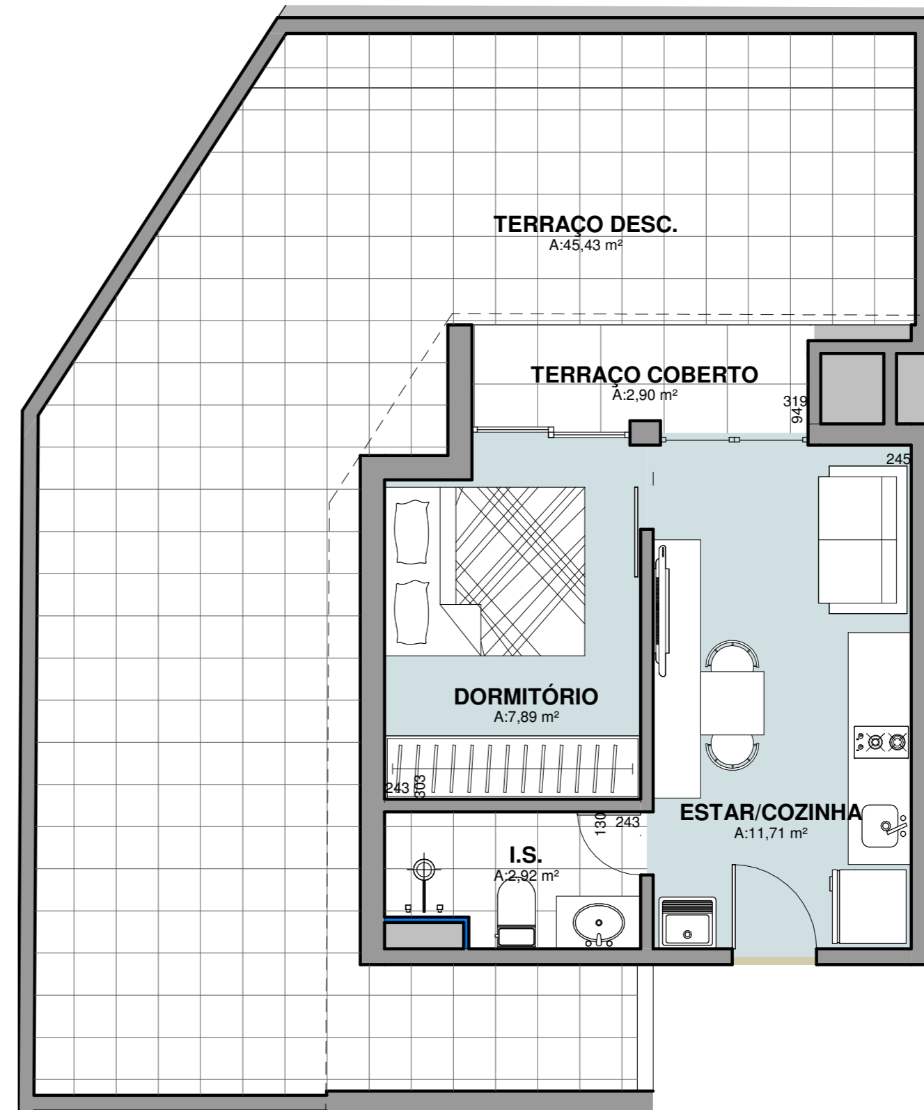
UN. TÉRREA - 109 ESCALA 1 : 50
